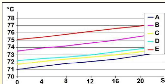
Temps de réponse à une élévation de température rapide à 6°C/min.
