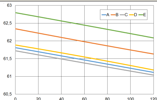
Temps de réponse à une baisse de température lente à 0.25°C/min
